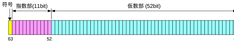
図 13.1 IEEE 754 による double のビット割り当て
