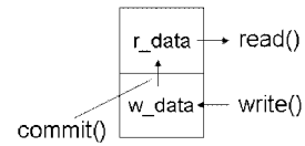
(b) バッファリングを行うレジスタ
