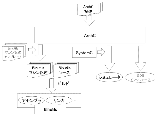
図 1 ArchC の処理の流れ
